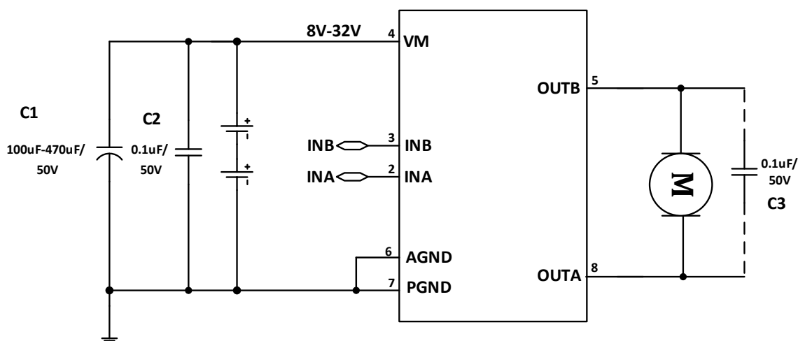
图 1 MX500HC 典型应用线路图
