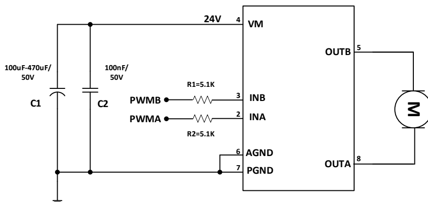
图 3 MX500HC 驱动风扇摇头电机应用线路图
