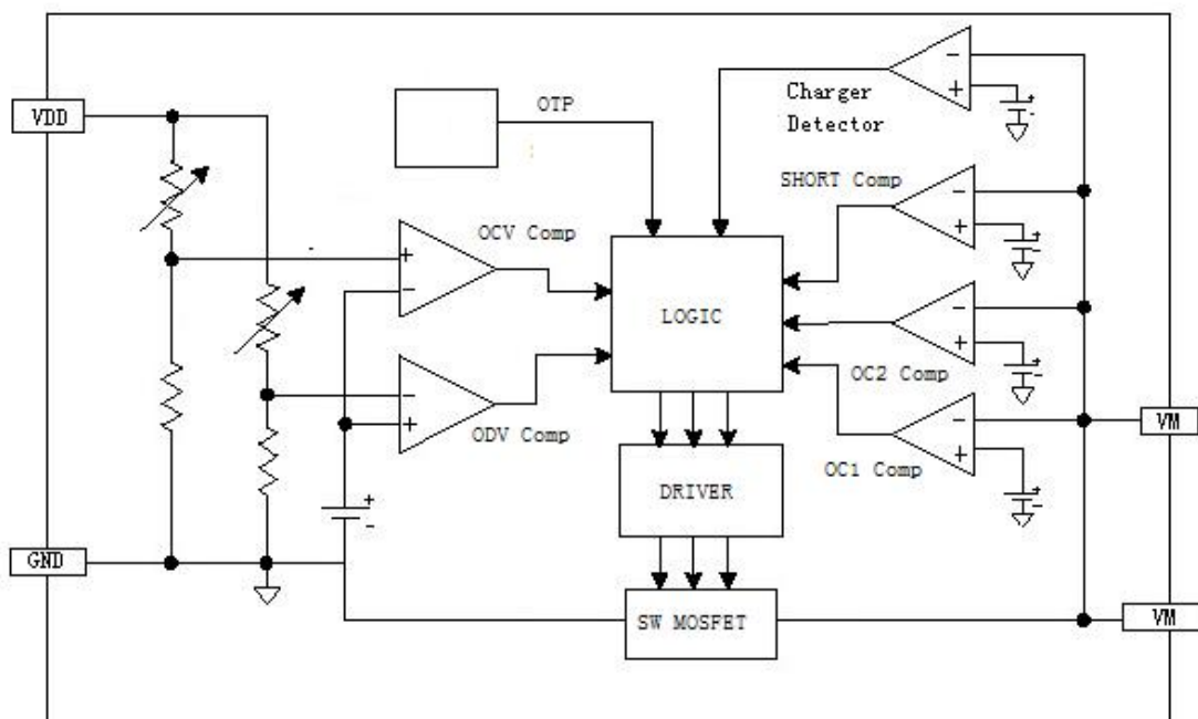
Figure 1. 原理图
