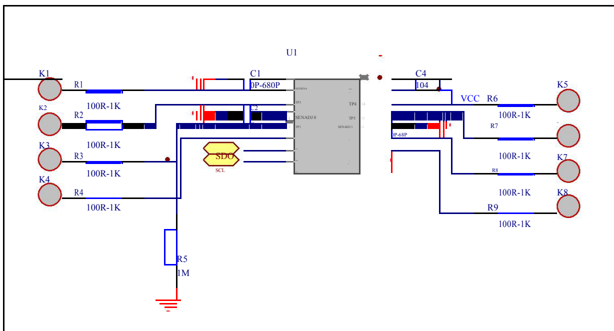
图 8-1 参考电路图
