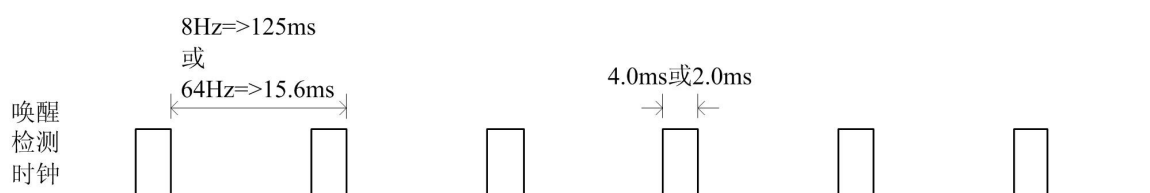
图 5-3 唤醒采样率和采样长度图
