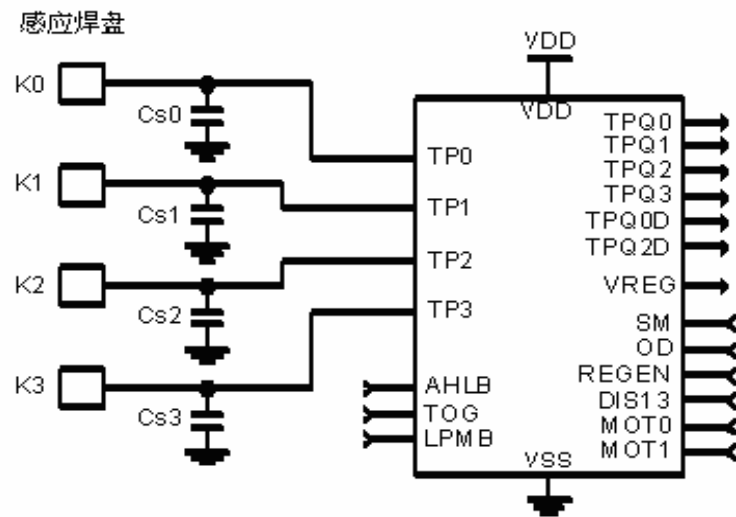
图 5-1 电容与各按键关系图
