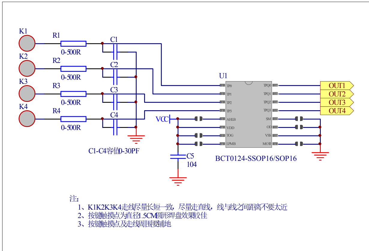
图 9-1 BCT0124-SOP16/SSOP16-4KEY 参考电路图
