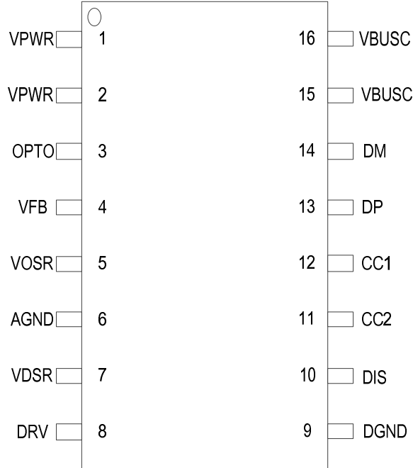
TSSOP16
