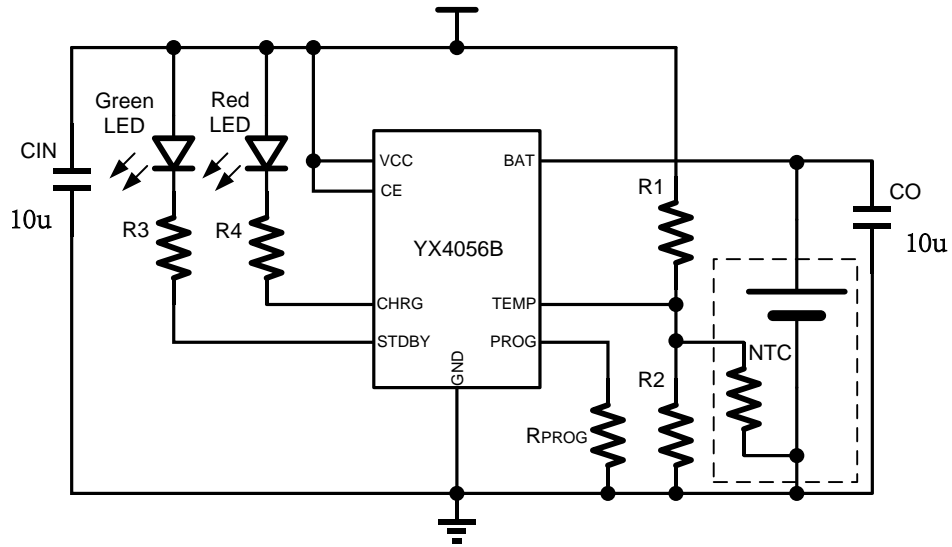
图 4. 典型应用电路
