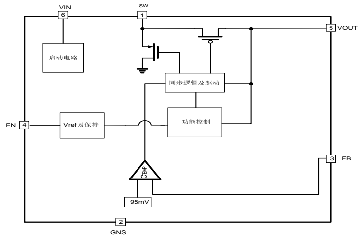
图 2. 内部框图
